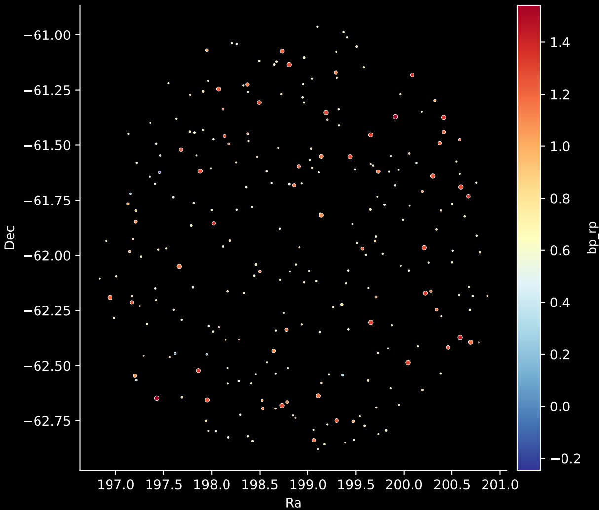
GALAH DR4 Field: [7143] Stars: 264
