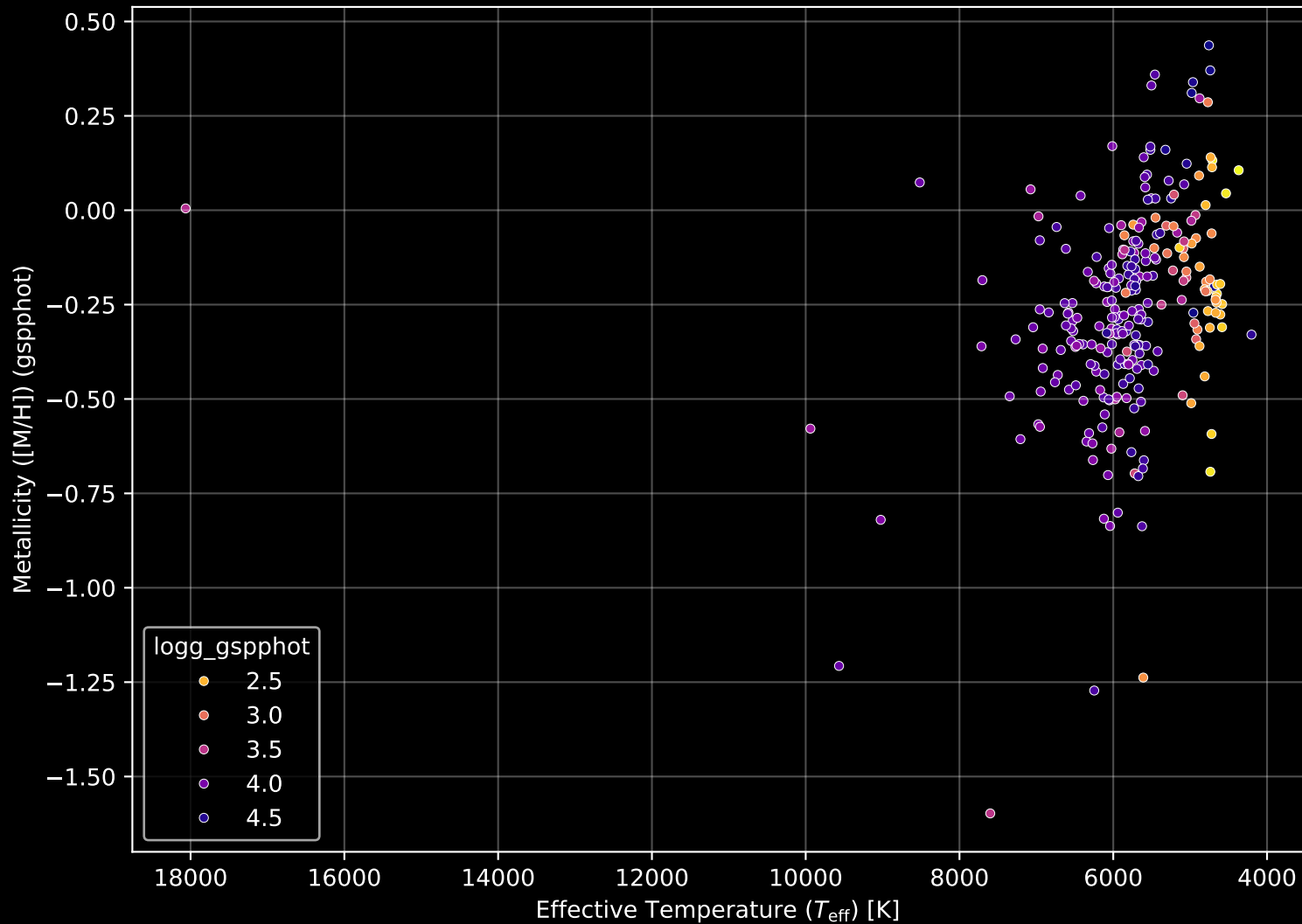
GALAH DR4 Field: [7143] Stellar Population Parameters (n= 264)
