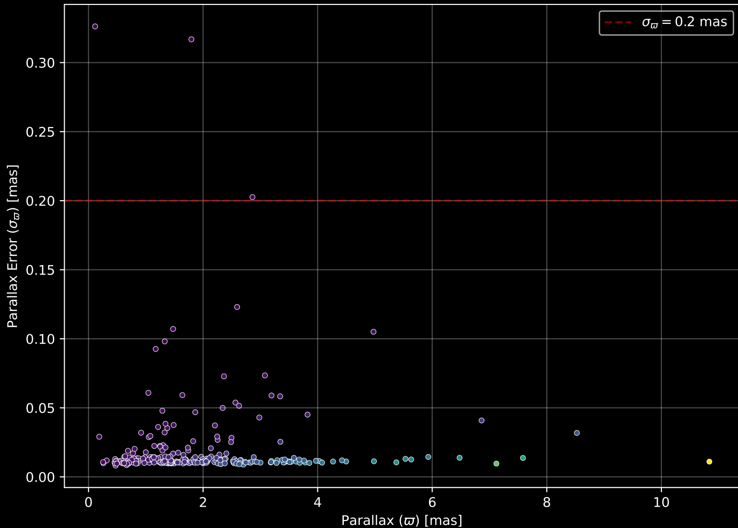
GALAH DR4 Field: [7143] Parallax Quality (n= 264)
