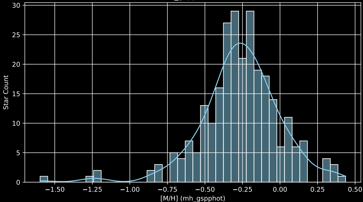
GALAH DR4 Field: [7143] [M/H] (mh_gspphot) (n= 264)
